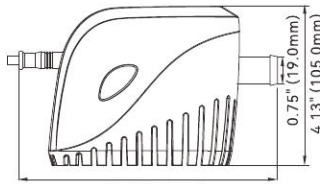
600 GPH-750 GPH
