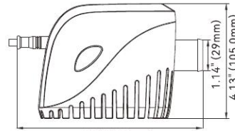
1100 GPH
