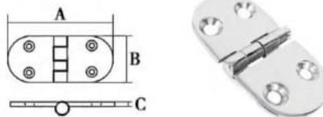
AlSi316 nerūdijančio plieno lietinis vyris
