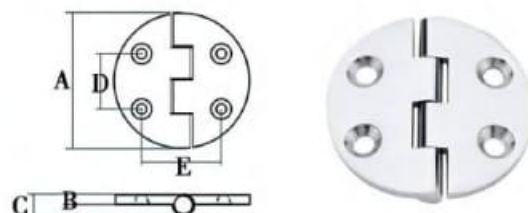
AlSi316 nerūdijančio plieno lietinis vyris
