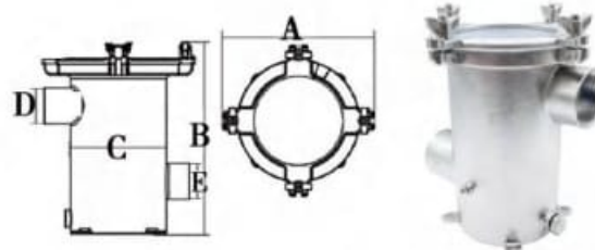
AISI316 nerūdijančio plieno vandens filtras
