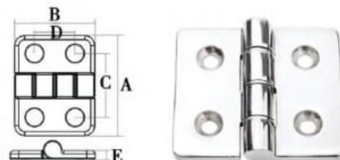
AISI316 nerūdijančio plieno tylus vyris
