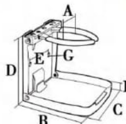
UPGRADED 316 nerūdijančio plieno sulankstomas puodelio laikiklis
