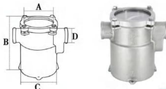
AISI316 nerūdijančio plieno vandens filtras
