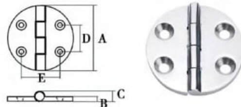
AlSi316 nerūdijančio plieno atvirkštinis apvalus lietinis vyris
