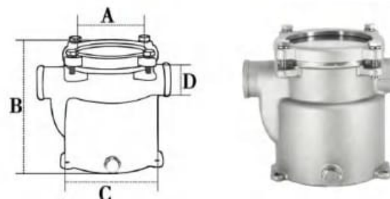
AISI316 nerūdijančio plieno vandens filtras
