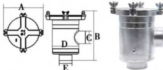
AISI316 nerūdijančio plieno vandens filtras
